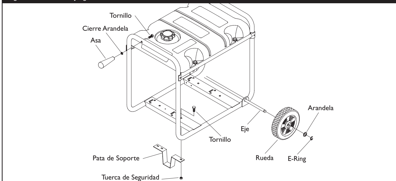
Figura 14 — Instale el Juego de Ruedas
